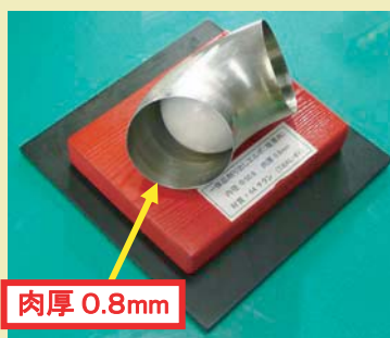
[2インチ64チタンエルボ薄肉タイプ] (内径より0.1mm 小さい球がエルボを通過)
