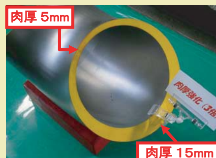
[エロージョン対応肉厚強化タイプ] (内径200mm 肉厚5~15mm)
